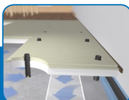
Passar alla golv oberoende av lutning och ojämnheter
